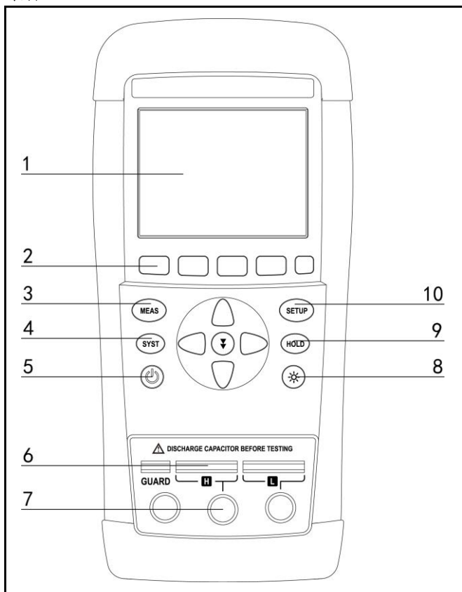
图 3-1 前面板
