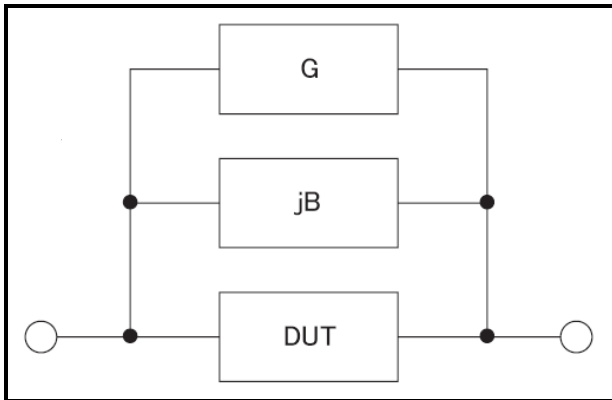
图 5-3 杂散导纳
