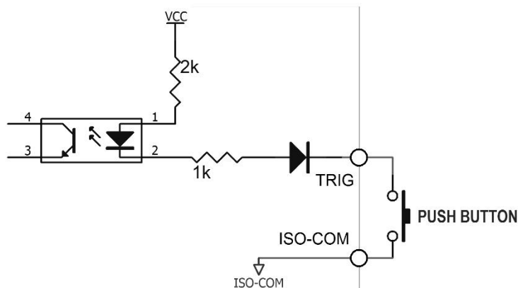
图 10-4 与开关的连接
