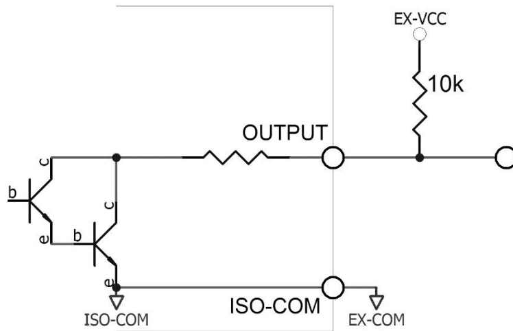
图 10-10 负逻辑输出
