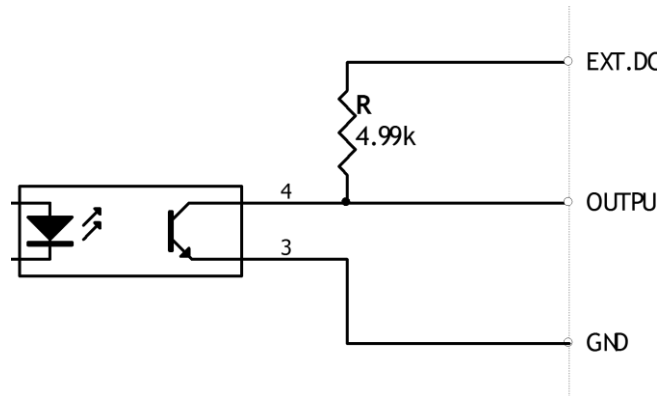
图 5-2 内部原理图
