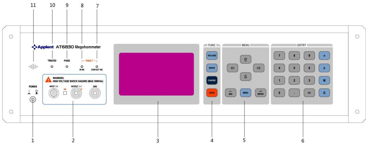
图 3-1 前面板
