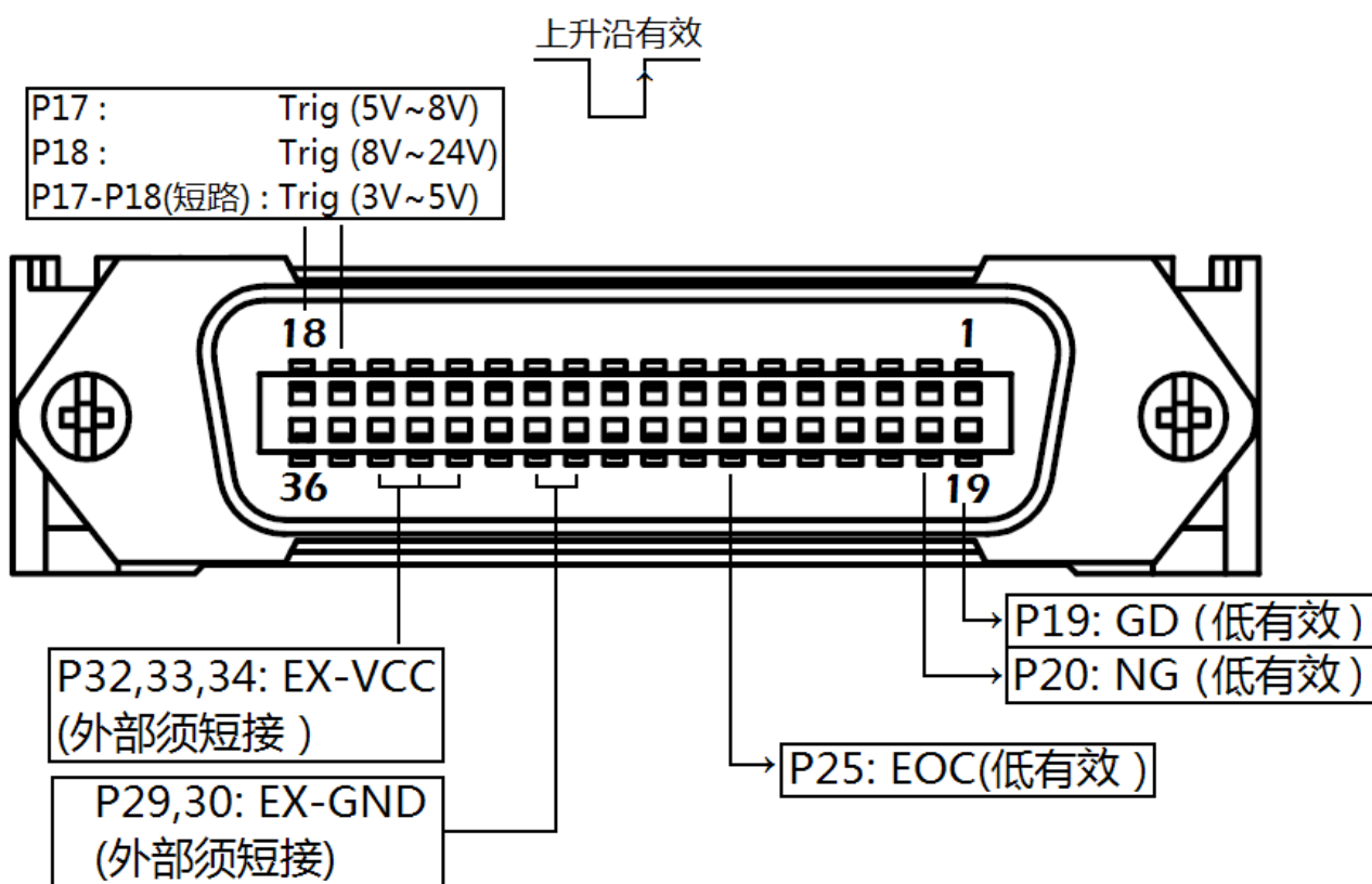
图 4-1 接线端子
