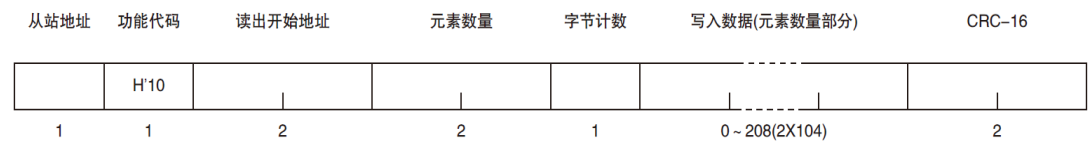
图 11-7 写入多个寄存器（0x10）
