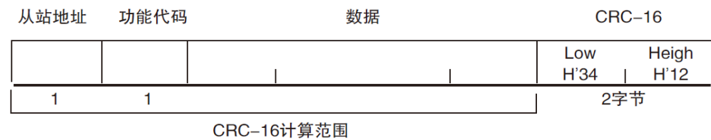
图 11-2 Modbus 附加 CRC-16 值
