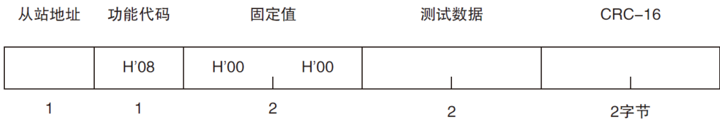
图 11-9 回波测试（0x08）
