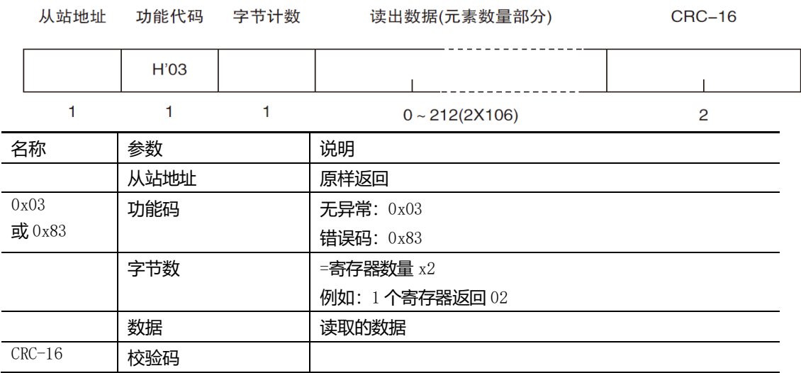
图 11-6 读出多个寄存器（0x03）响应帧
