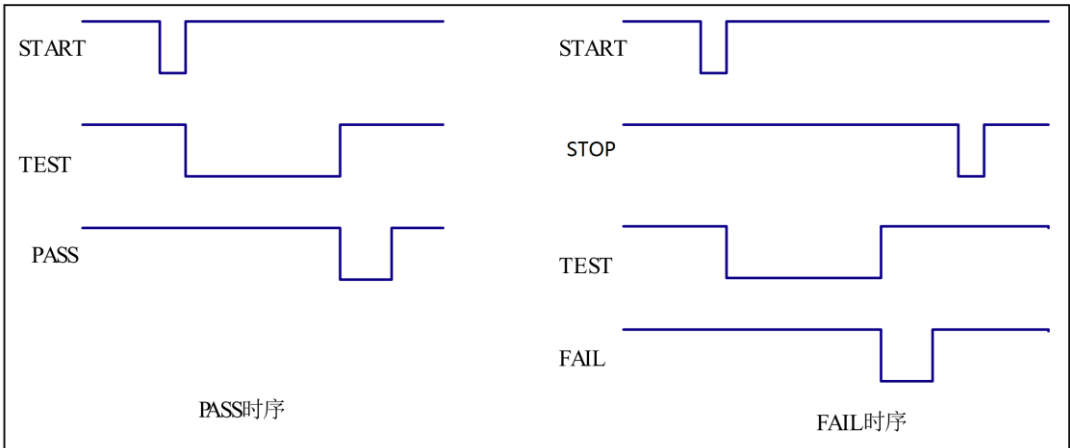
图 8-3 PLC 时序图
